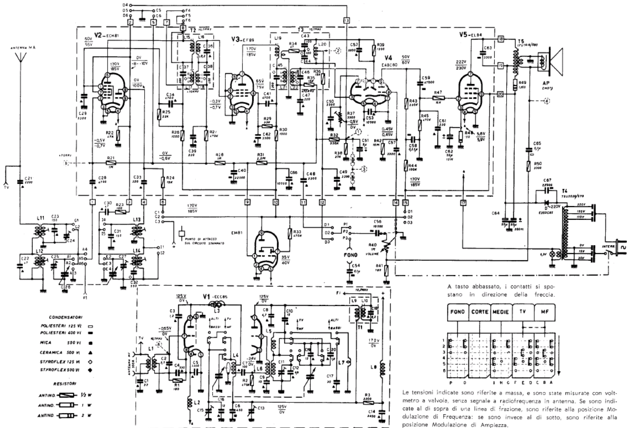
RADIORICEVITORE PHONOLA Mod. «Phonoletta» PH 687 C
